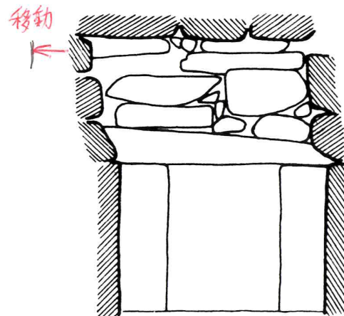
34 横断面図
