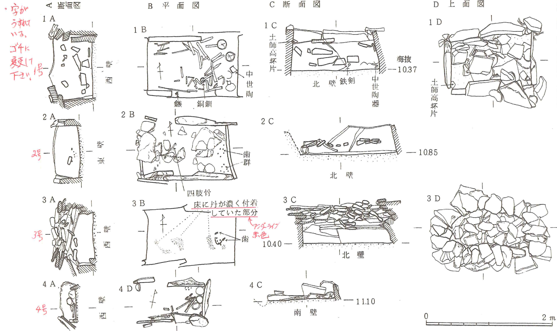
14QG 第187図 妻の鼻墳墓群 1. 2. 3. 4号 地下式石室墓実測図 (報告書13頁参照)
